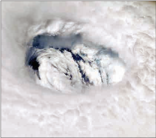
اقیانوس طلسم- تصویری از طوفان دوریان که توسط نیک‌هاگ، یکی از فضانوردان ناسا مستقر در ایستگاه فضایی بین‌المللی گرفته شده‌است.
